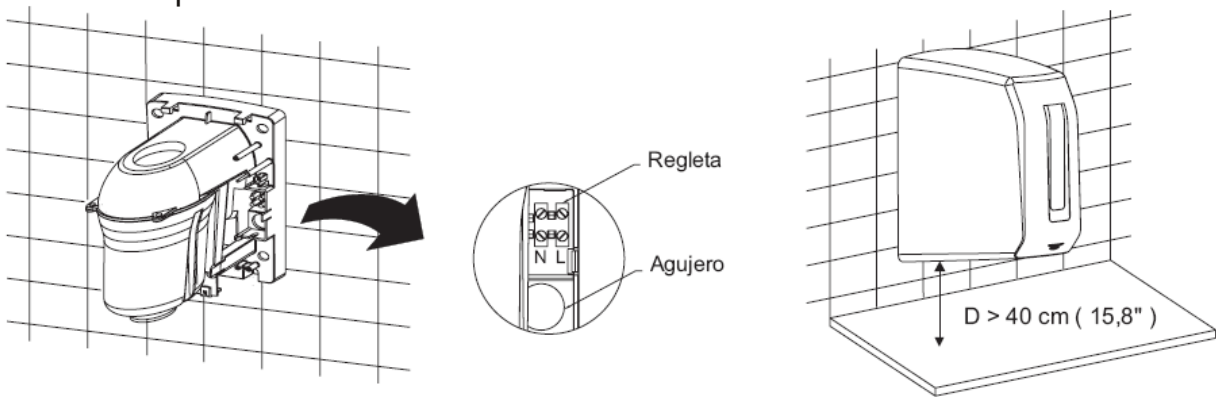
Ubicación regleta y agujero Ø 22 mm ( Ø 0.87" ) de entrada cables
