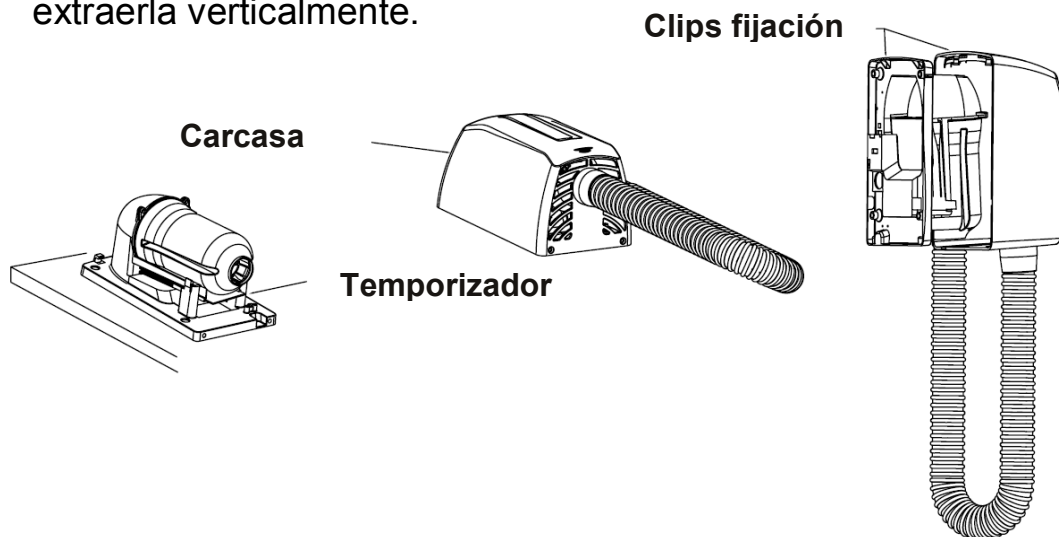
Detalle clips fijación base-carcasa
