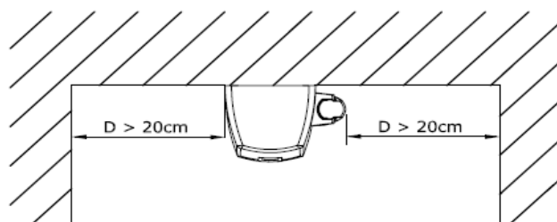
Distance minimale sèche-cheveux/étagère et sèche-cheveux/murs
