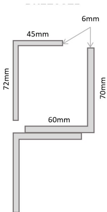
DIMENSIONS
