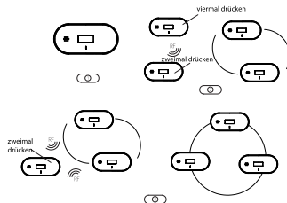
Abbildung 5-1 Gerät verbinden
