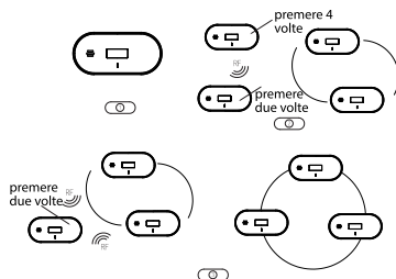
Figura 5-1 Interconnessione dispositivo
