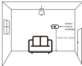
Abbildung 7-3 Installation des Melders in einem Wohnzimmer ohne eines mit Brennstoff betriebenen Geräts
