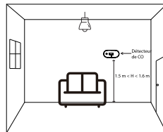
Figure 7-3 Installation dans une salle de jour avec un appareil à combustible
