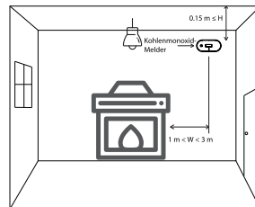
Abbildung 7-2 Installation in einem Raum, in dem sich ein mit Brennstoff betriebenes Gerät befindet
