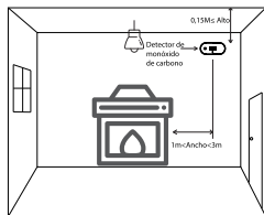
Figura 7-2 Instalación en una habitación con un aparato que quema combustible
