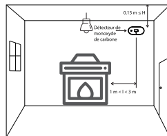
Figure 7-2 Installation dans une pièce avec un appareil à combustible
