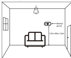
Figura 7-3 Instalación en una sala de estar sin un aparato que quema combustible
