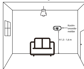
Afbeelding 7-3 Installatie in een woonkamer zonder een verbrandingstoestel
