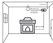
Figura 7-2 Installazione in una stanza con dispositivi a combustione
