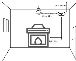
Afbeelding 7-2 Installatie in een ruimte met een verbrandingstoestel
