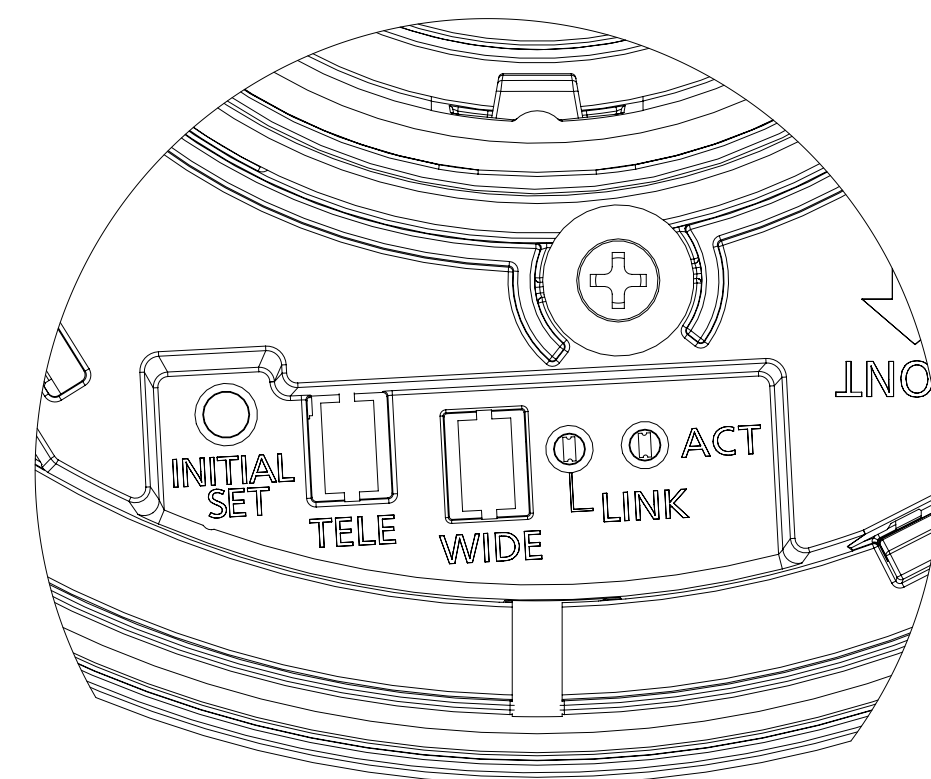
Detail B S=2 : 1
